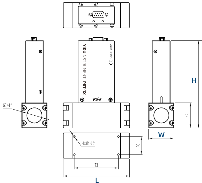
500SLPM 尺寸图
