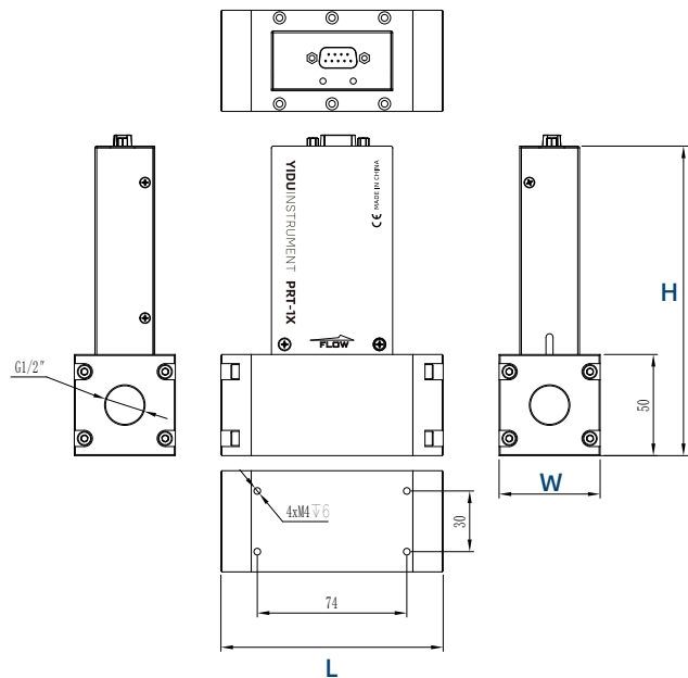
1000SLPM 尺寸图
